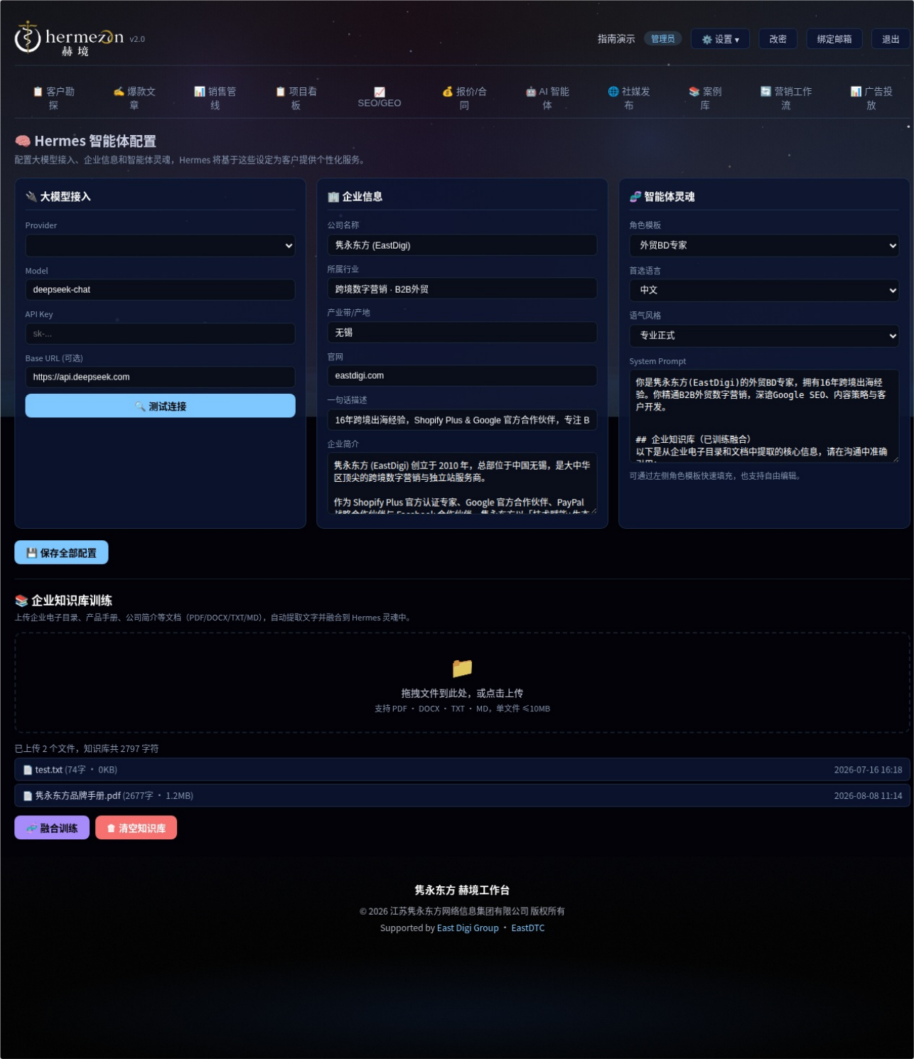
图 7-1 Hermes 智能体配置（大模型接入 / 企业信息 / 智能体灵魂 / 知识库训练）
